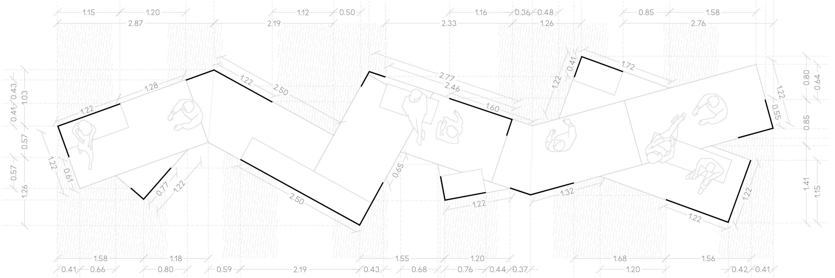
DESPIECE DE LOS TABLEROS DURAPLY
