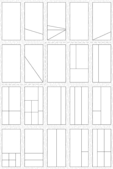
DESPIECE DE LOS TABLEROS DURAPLY
